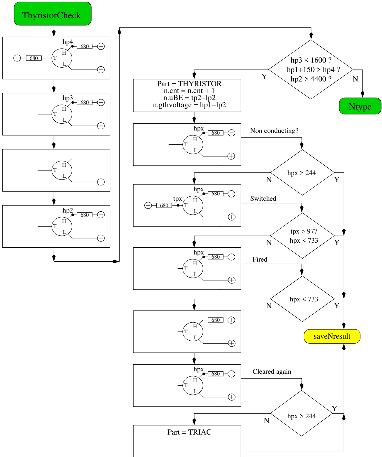
Abbildung 5.10. Ablaufplan der Transistorprüfung Teil 3, Thyristor und Triac
