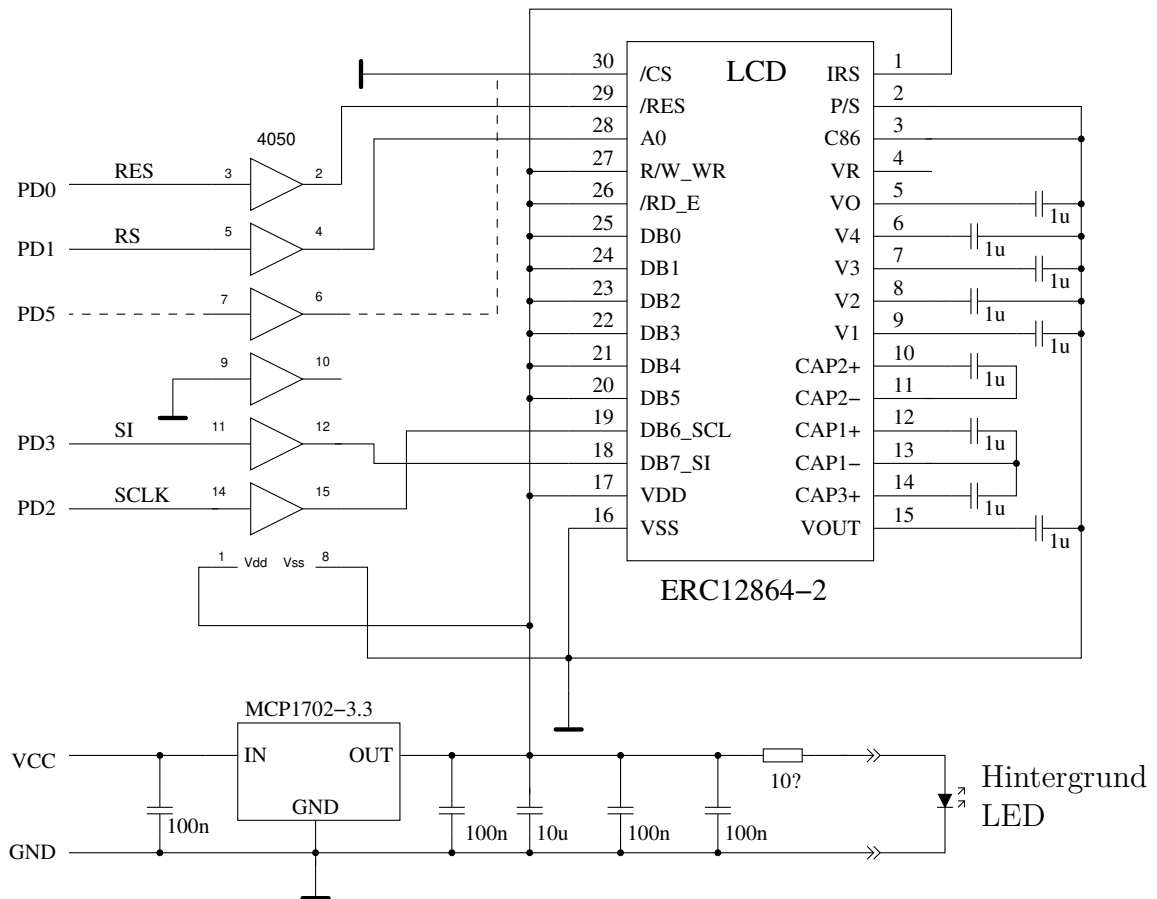
Abbildung 2.9. Anschluss eines graphischen Displays mit ST7565 Controller
