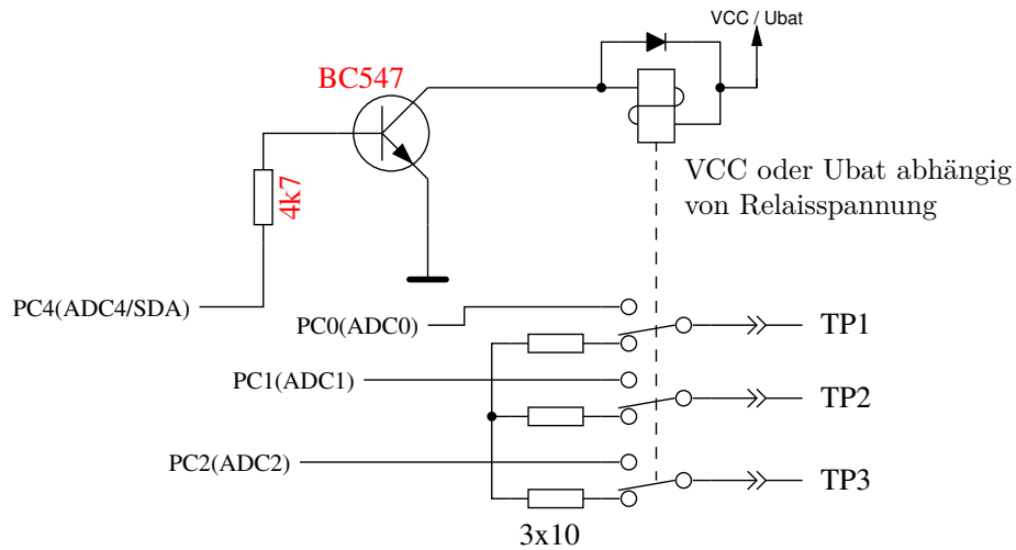
Abbildung 2.3. Verbesserter Schutz mit Relais
