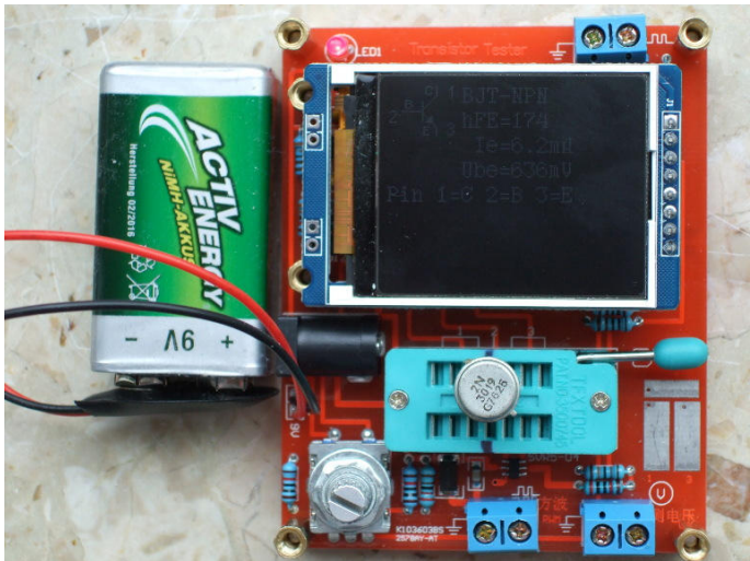
(a) zusammgebaut
