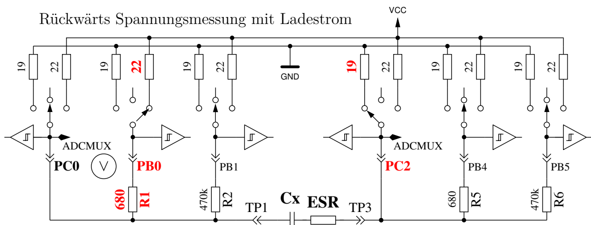
Abbildung 5.40. Vereinfachte ESR-Messung eines Kondensators
