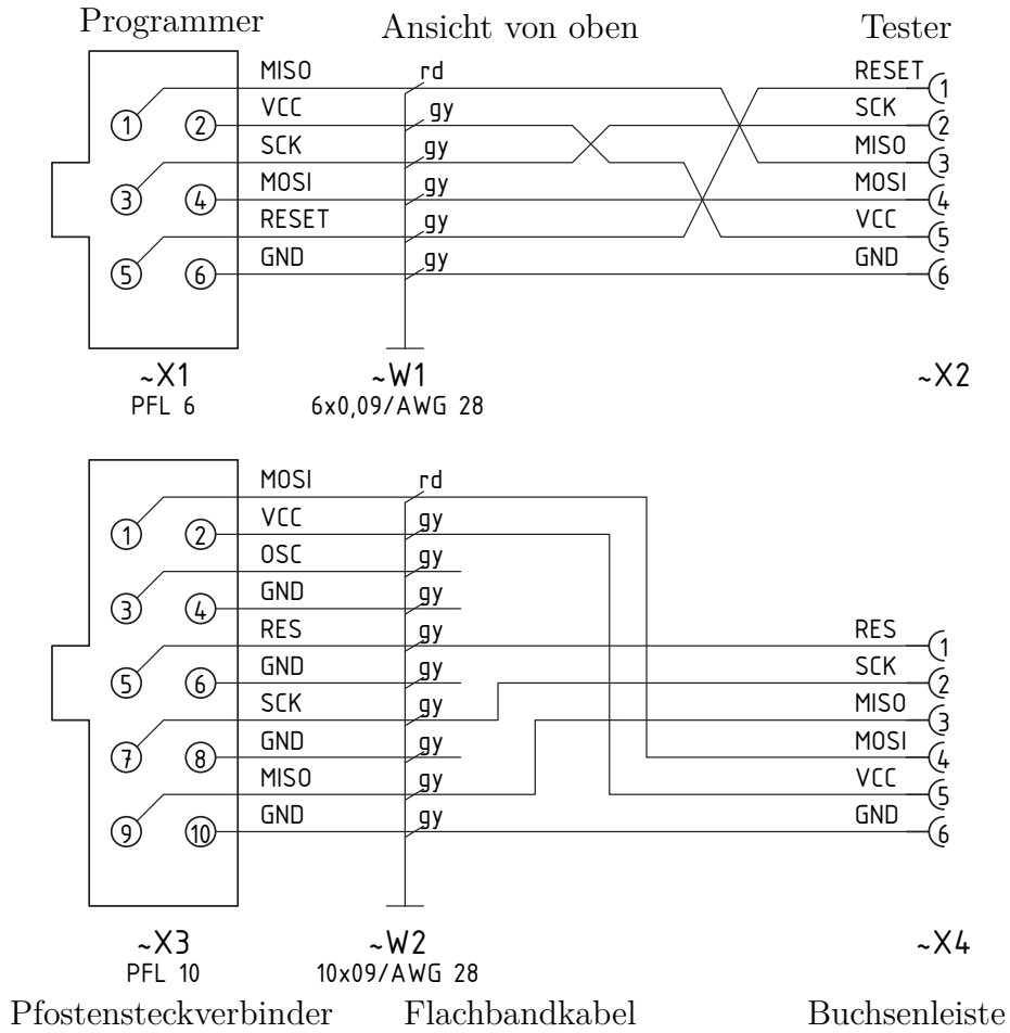
Abbildung 2.28. 6 und 10 Pol Kabel für die Programmierung
