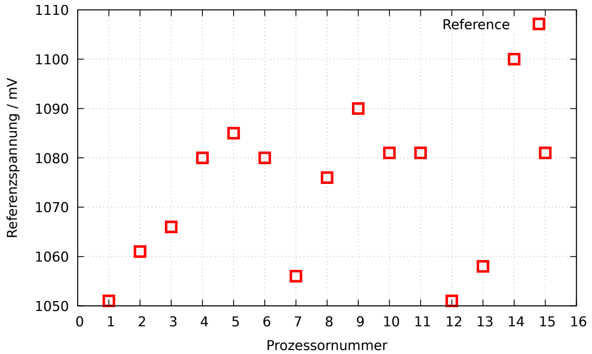
Abbildung 5.69. Selbsttest: Referenz-Spannungen
