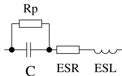
Abbildung 5.31. Kondensator-Ersatzschaltbild
