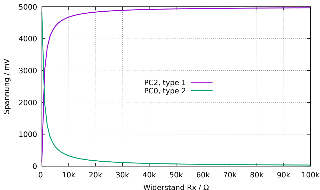
Abbildung 5.13. Spannung von Type 1 und Type 2 mit Messwiderstand 680\Omega
