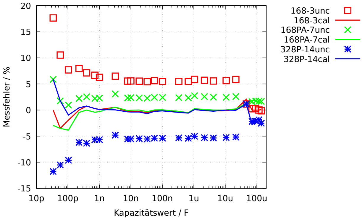
Abbildung 5.60. Kondensator-Messfehler von drei ATmega, vor und nach der Kalibrierung
