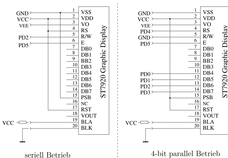
Abbildung 2.11. Anschluss eines Displays mit ST7920 Controller
