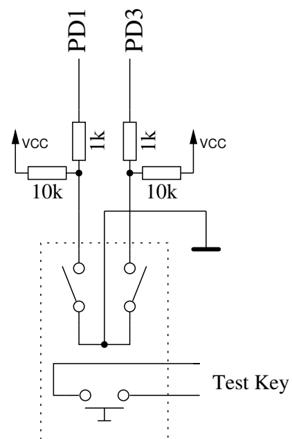
Abbildung 2.6. Impulsdrehgeber-Erweiterung
