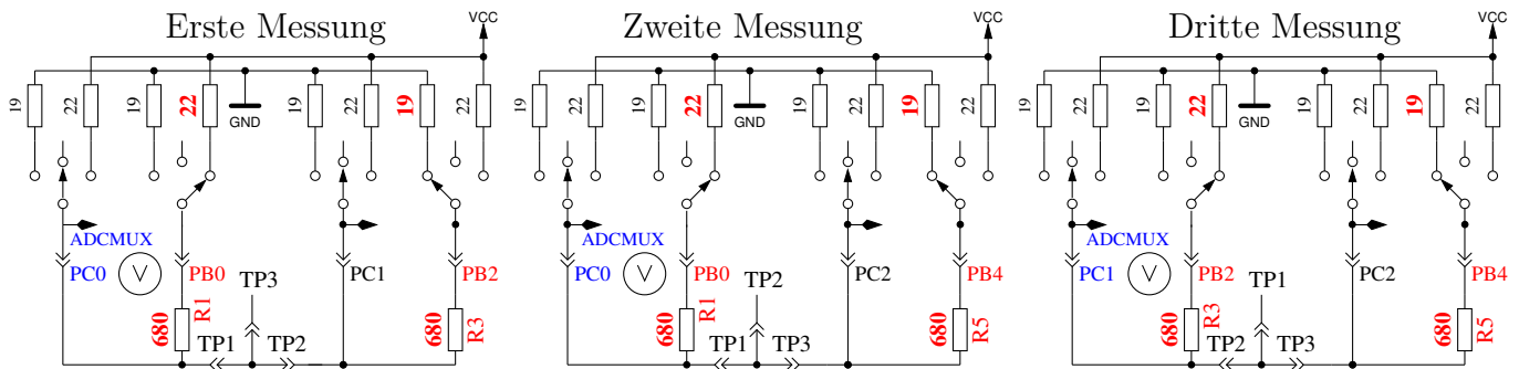
Abbildung 5.65. Vergleich der 680\Omega -Widerstände
