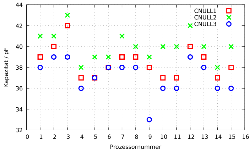
Abbildung 5.73. Selbsttest: Nullwert der Kapazitätsmessung
